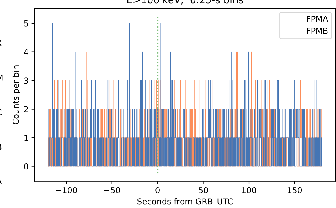
E>100 keV, 0.25-s bins
