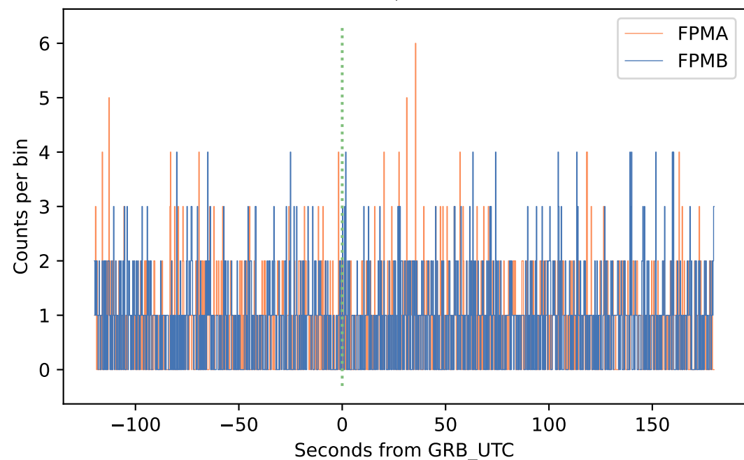
E>100 keV, 0.25-s bins
