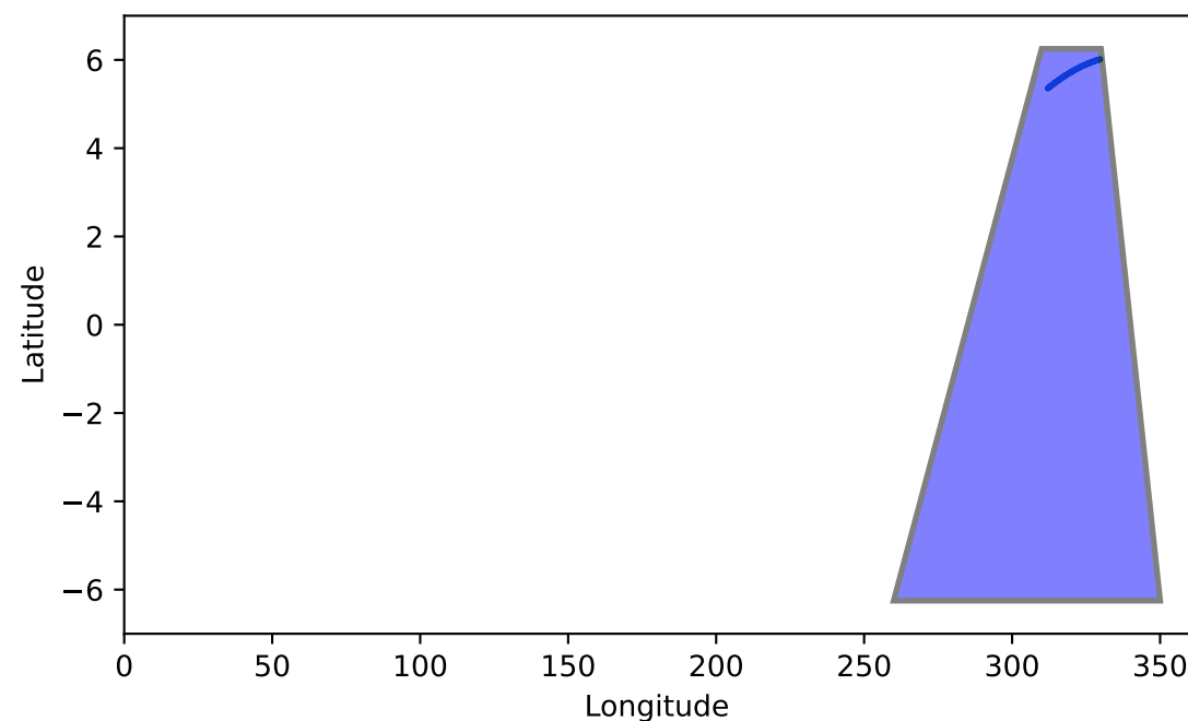
E>100 keV, 5.00-s bins
