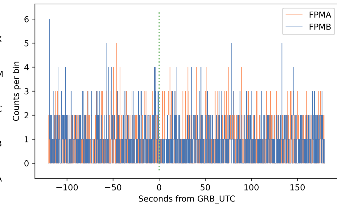
E>100 keV, 0.25-s bins
