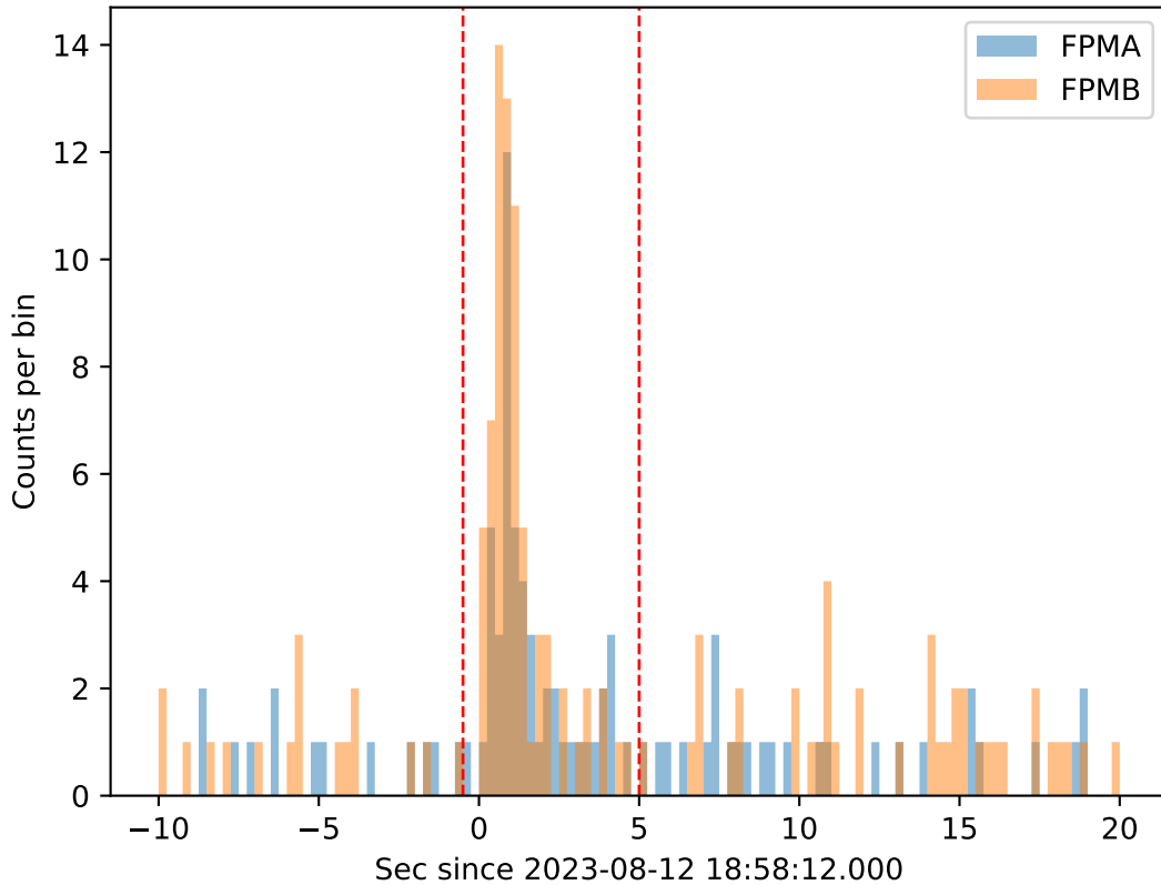
GRB230812B 40-300 keV CZT Lightcurve, 0.25-s bins
