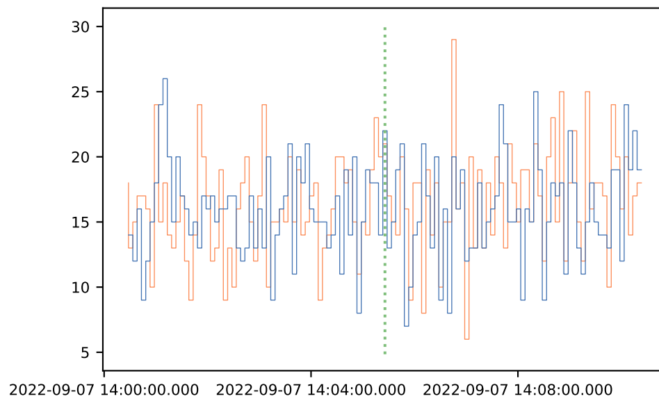
E>100 keV, 0.25-s bins
