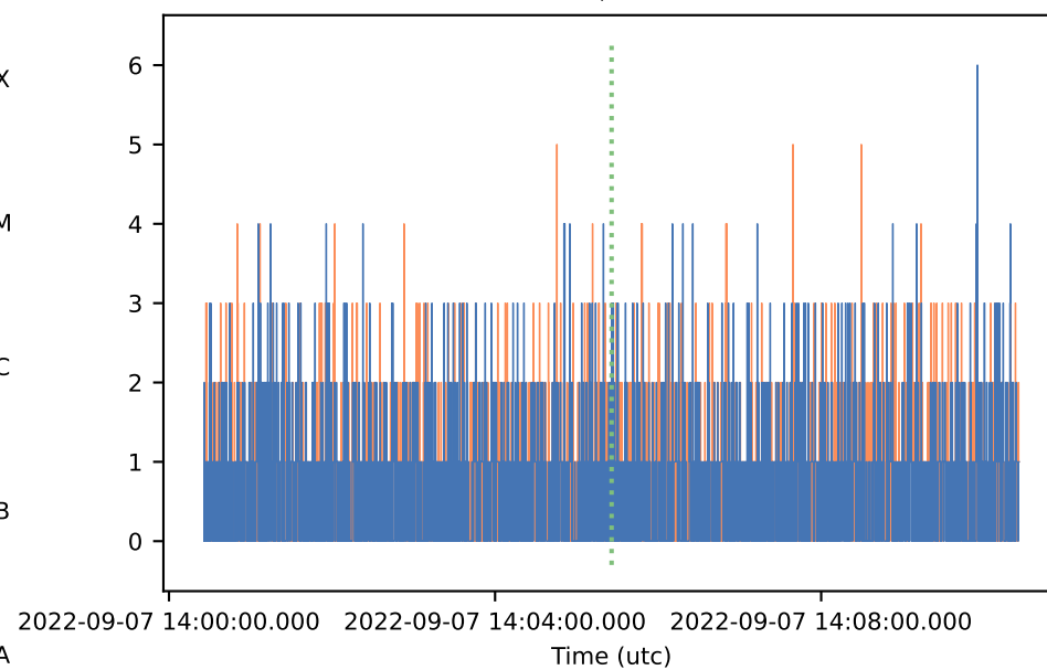
E>100 keV, 0.25-s bins
