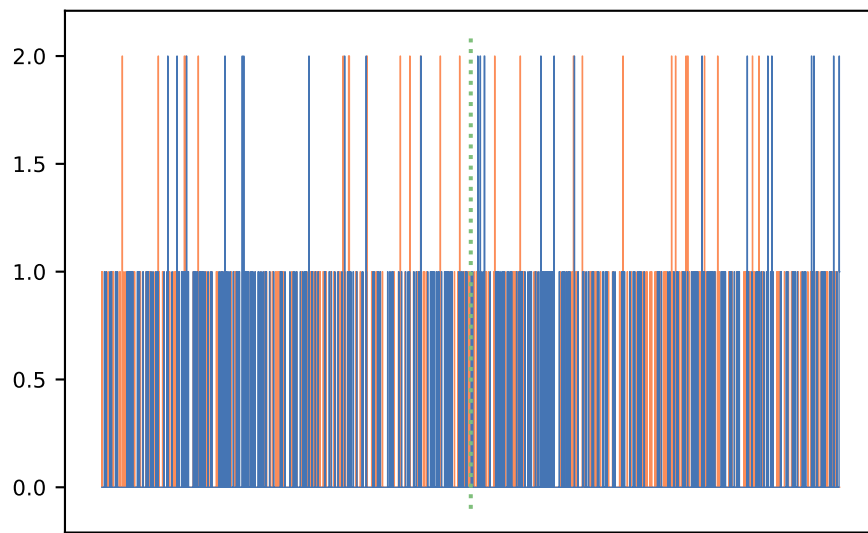
E>100 keV, 0.25-s bins
