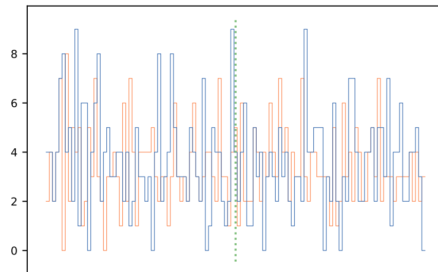
E>100 keV, 5.00-s bins
