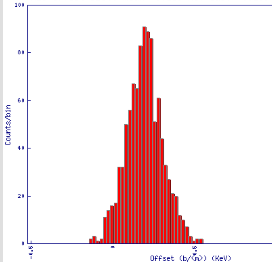
H25 Offset Dist: mean= 0.189 KeV sdev= 0.109
