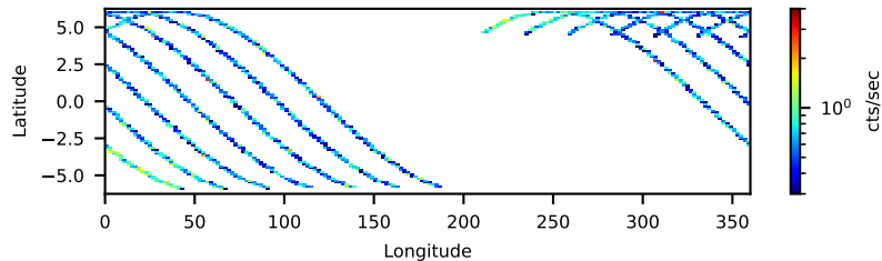
--saacalc=1 -saamode=OPTIMIZED --tentacle=yes 21.25-ks, 100%
