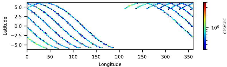
--saacalc=1 -saamode=OPTIMIZED --tentacle=no 21.25-ks, 100%
