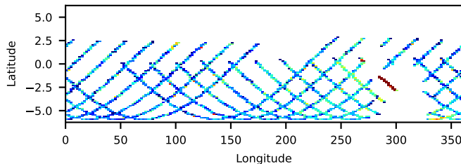
--saacalc=1 -saamode=OPTIMIZED --tentacle=yes 34.58-ks, 94%
