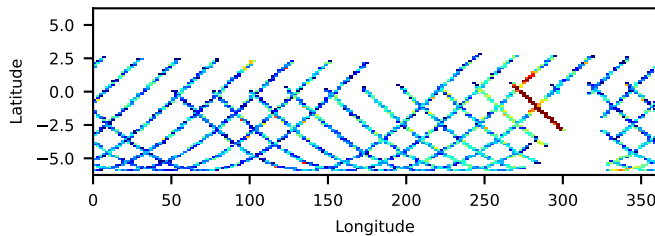
--saacalc=1 -saamode=OPTIMIZED --tentacle=no 35.23-ks, 96%
