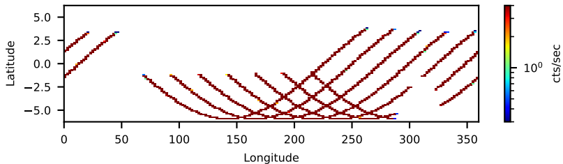
--saacalc=1 -saamode=OPTIMIZED --tentacle=yes 12.81-ks, 100%
