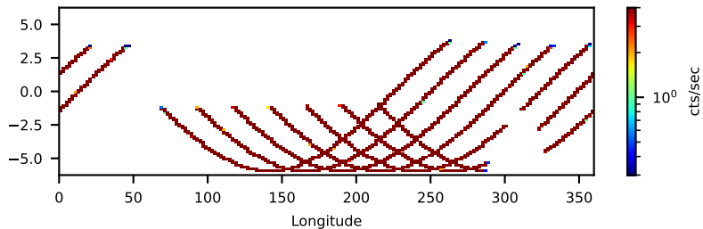
--saacalc=3 -saamode=OPTIMIZED --tentacle=yes 12.81-ks, 100%
