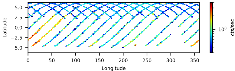
--saacalc=1 -saamode=OPTIMIZED --tentacle=yes 41.82-ks, 99%
