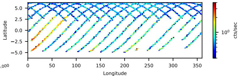
--saacalc=2 -saamode=OPTIMIZED --tentacle=yes 41.68-ks, 99%
