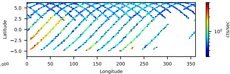
--saacalc=3 --saamode=STRICT --tentacle=yes 38.82-ks, 92%
