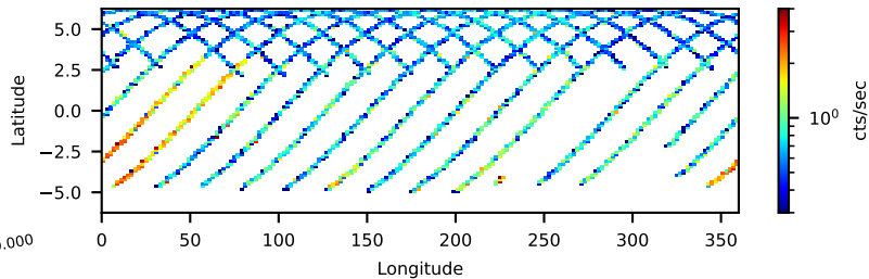
--saacalc=3 -saamode=OPTIMIZED --tentacle=no 41.68-ks, 99%
