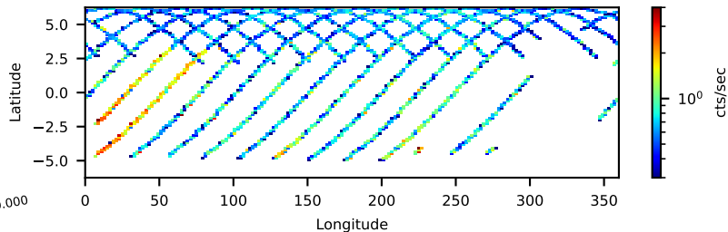
--saacalc=3 --saamode=STRICT --tentacle=yes 38.82-ks, 92%
