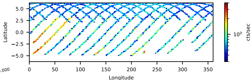
--saacalc=2 -saamode=OPTIMIZED --tentacle=yes 41.68-ks, 99%
