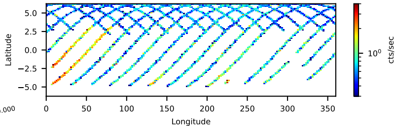
--saacalc=3 -saamode=OPTIMIZED --tentacle=yes 41.68-ks, 99%
