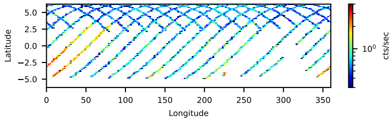
--saacalc=1 -saamode=OPTIMIZED --tentacle=no 41.82-ks, 99%
