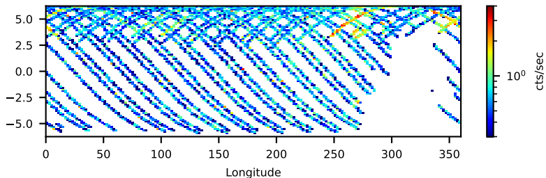
--saacalc=3 -saamode=STRICT --tentacle=yes 77.65-ks, 88%
