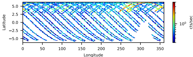
--saacalc=1 -saamode=OPTIMIZED --tentacle=yes 86.54-ks, 98%
