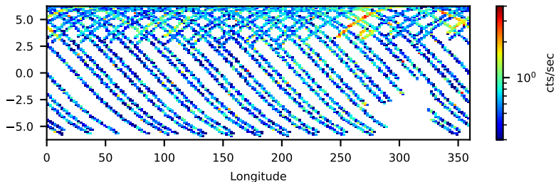
--saacalc=2 -saamode=OPTIMIZED --tentacle=yes 84.00-ks, 96%
