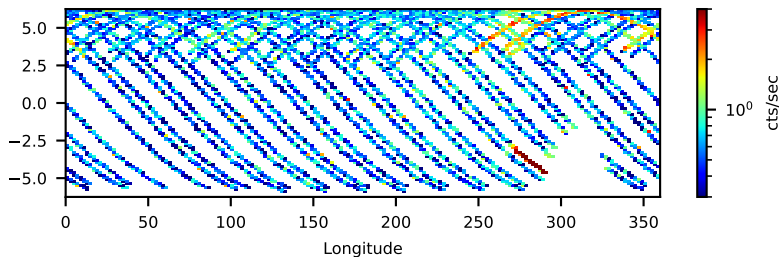
--saacalc=2 -saamode=OPTIMIZED --tentacle=no 86.28-ks, 98%
