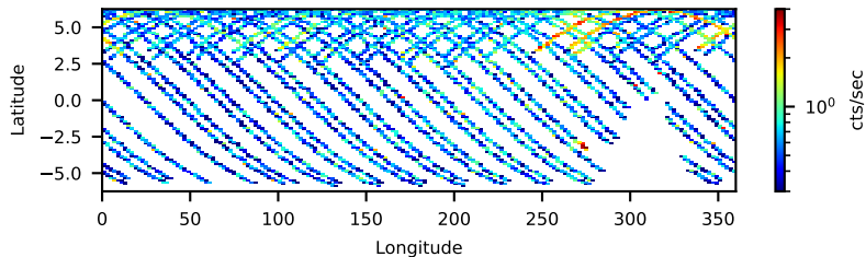
--saacalc=1 -saamode=OPTIMIZED --tentacle=no 86.95-ks, 99%
