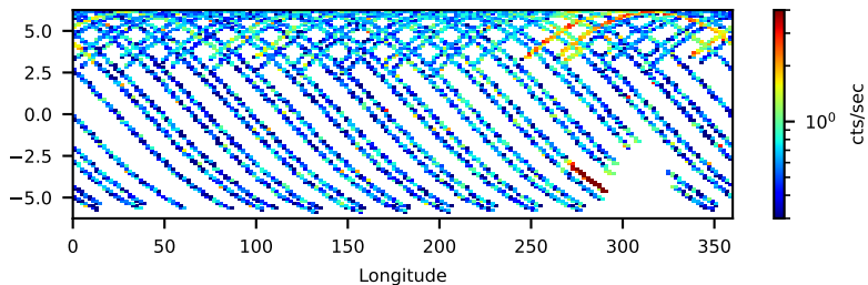
--saacalc=3 -saamode=OPTIMIZED --tentacle=no 86.19-ks, 98%
