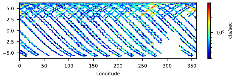
--saacalc=3 -saamode=OPTIMIZED --tentacle=yes 83.41-ks, 95%
