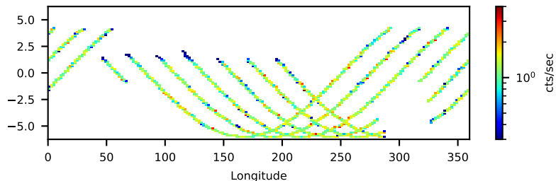
--saacalc=2 -saamode=OPTIMIZED --tentacle=yes 18.61-ks, 99%
