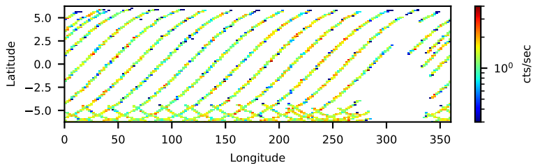
--saacalc=1 -saamode=OPTIMIZED --tentacle=yes 40.01-ks, 94%
