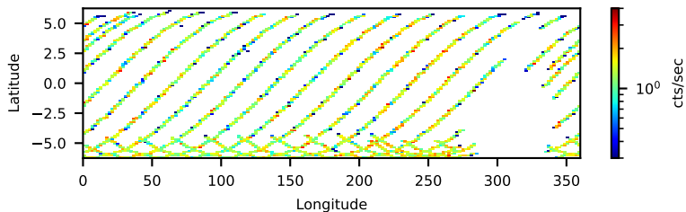
--saacalc=1 -saamode=OPTIMIZED --tentacle=no 40.01-ks, 94%
