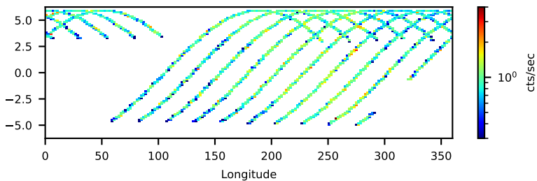
--saacalc=3 -saamode=STRICT --tentacle=no 26.00-ks, 90%
