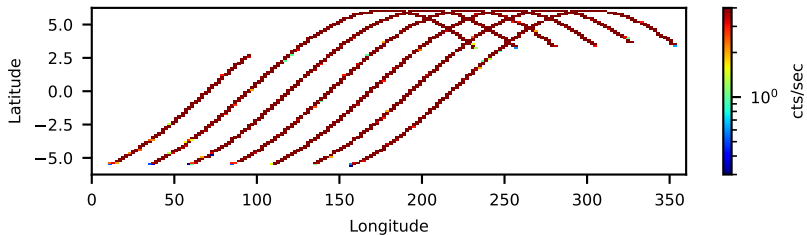
--saacalc=1 -saamode=OPTIMIZED --tentacle=yes 19.69-ks, 100%
