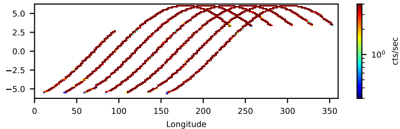
--saacalc=3 -saamode=OPTIMIZED --tentacle=no 19.72-ks, 100%
