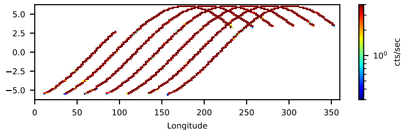
--saacalc=2 -saamode=OPTIMIZED --tentacle=yes 19.72-ks, 100%
