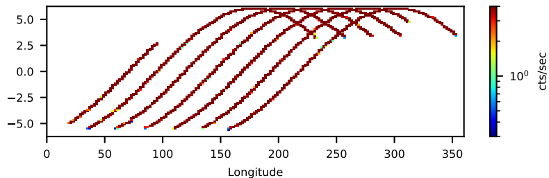
--saacalc=3 -saamode=STRICT --tentacle=yes 19.36-ks, 98%
