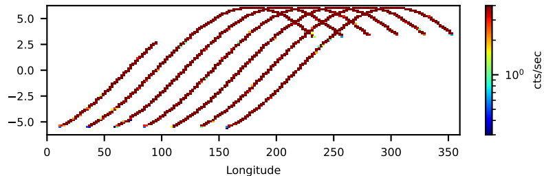
--saacalc=3 -saamode=OPTIMIZED --tentacle=yes 19.72-ks, 100%
