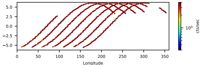
--saacalc=1 -saamode=STRICT --tentacle=yes 18.99-ks, 96%
