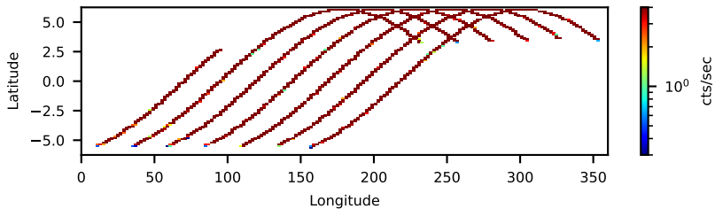
--saacalc=1 -saamode=OPTIMIZED --tentacle=no 19.69-ks, 100%
