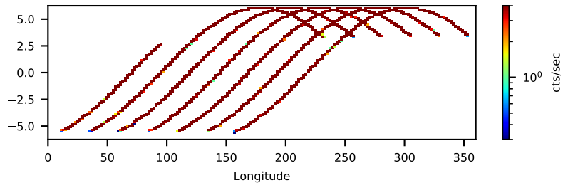
--saacalc=1 -saamode=STRICT --tentacle=no 18.99-ks, 96%
