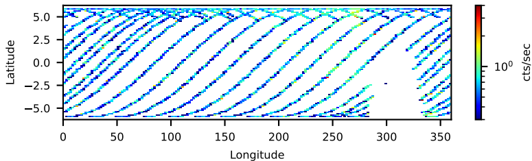
--saacalc=1 -saamode=OPTIMIZED --tentacle=yes 54.52-ks, 98%
