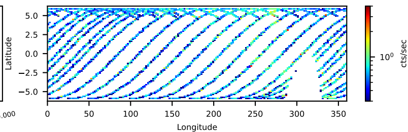
--saacalc=3 -saamode=OPTIMIZED --tentacle=no 54.38-ks, 98%
