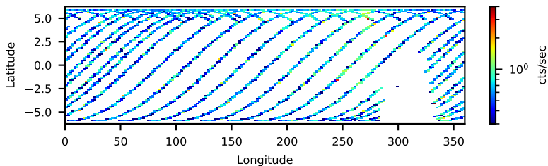
--saacalc=1 -saamode=OPTIMIZED --tentacle=no 54.52-ks, 98%
