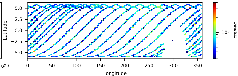
--saacalc=3 -saamode=OPTIMIZED --tentacle=yes 53.45-ks, 96%
