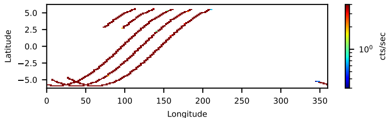
--saacalc=1 -saamode=OPTIMIZED --tentacle=yes 4.10-ks, 100%
