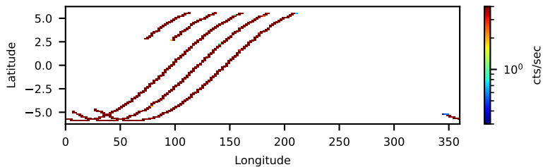
--saacalc=1 -saamode=OPTIMIZED --tentacle=no 4.10-ks, 100%
