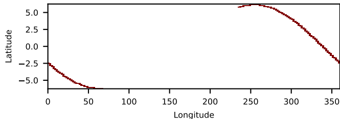
--saacalc=1 -saamode=OPTIMIZED --tentacle=yes 2.70-ks, 100%
