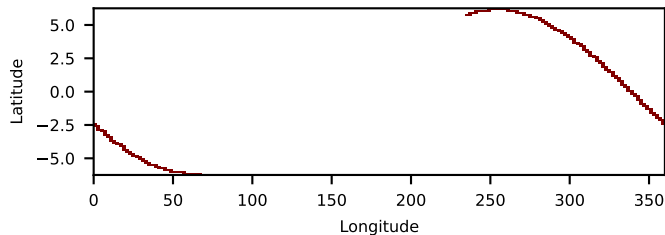
--saacalc=1 -saamode=OPTIMIZED --tentacle=no 2.70-ks, 100%
