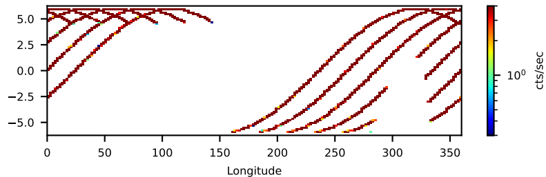
--saacalc=2 -saamode=OPTIMIZED --tentacle=yes 15.44-ks, 100%
