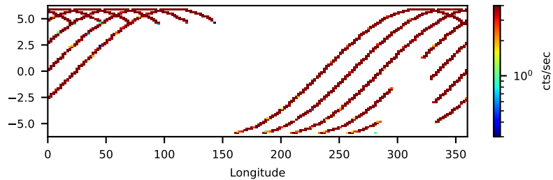
--saacalc=2 -saamode=OPTIMIZED --tentacle=no 15.44-ks, 100%
