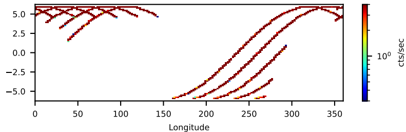
--saacalc=3 -saamode=STRICT --tentacle=yes 11.92-ks, 77%
