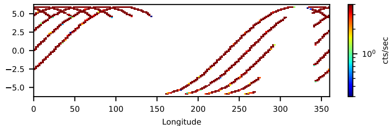
--saacalc=1 -saamode=STRICT --tentacle=yes 13.25-ks, 86%
