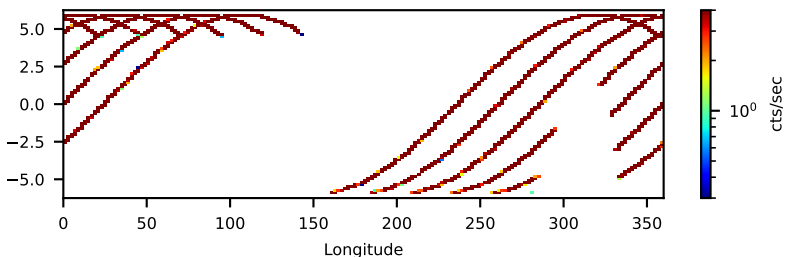
--saacalc=3 -saamode=OPTIMIZED --tentacle=yes 15.44-ks, 100%
