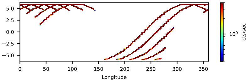
--saacalc=2 -saamode=STRICT --tentacle=yes 11.92-ks, 77%
