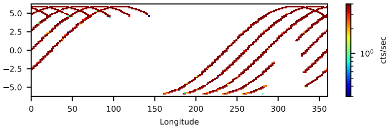
--saacalc=2 -saamode=STRICT --tentacle=no 11.92-ks, 77%
