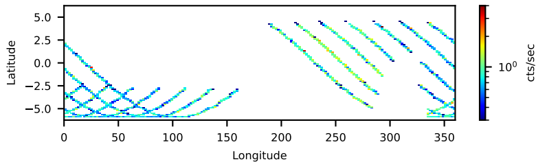
--saacalc=1 -saamode=OPTIMIZED --tentacle=no 17.90-ks, 98%
