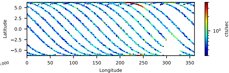
--saacalc=1 -saamode=STRICT --tentacle=no 38.00-ks, 93%
