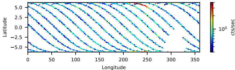
--saacalc=1 -saamode=OPTIMIZED --tentacle=no 40.44-ks, 99%
