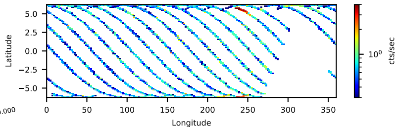
--saacalc=2 -saamode=STRICT --tentacle=yes 36.81-ks, 90%
