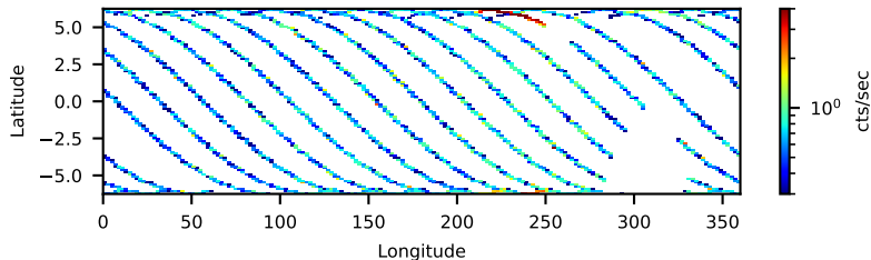
--saacalc=1 -saamode=OPTIMIZED --tentacle=yes 40.20-ks, 98%
