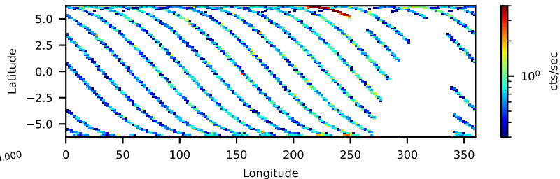
--saacalc=1 -saamode=STRICT --tentacle=yes 37.75-ks, 92%
