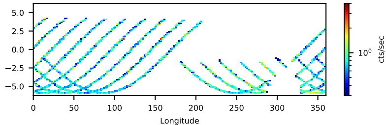
--saacalc=3 -saamode=OPTIMIZED --tentacle=no 24.23-ks, 100%
