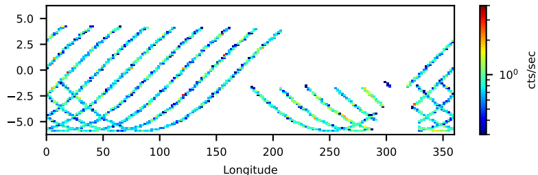
--saacalc=3 -saamode=OPTIMIZED --tentacle=yes 24.15-ks, 100%
