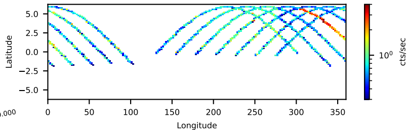
--saacalc=3 -saamode=OPTIMIZED --tentacle=yes 19.71-ks, 97%
