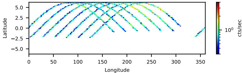
--saacalc=1 -saamode=OPTIMIZED --tentacle=no 21.57-ks, 99%
