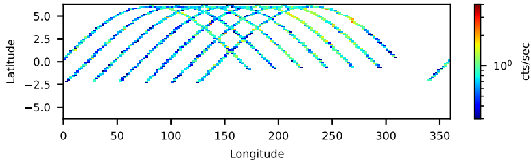
--saacalc=1 -saamode=OPTIMIZED --tentacle=yes 21.57-ks, 99%
