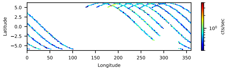
--saacalc=1 -saamode=OPTIMIZED --tentacle=no 19.06-ks, 97%
