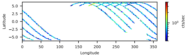
--saacalc=1 -saamode=OPTIMIZED --tentacle=yes 19.06-ks, 97%
