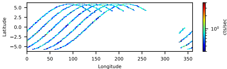
--saacalc=1 -saamode=OPTIMIZED --tentacle=no 18.50-ks, 99%
