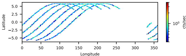
--saacalc=1 -saamode=OPTIMIZED --tentacle=yes 18.50-ks, 99%
