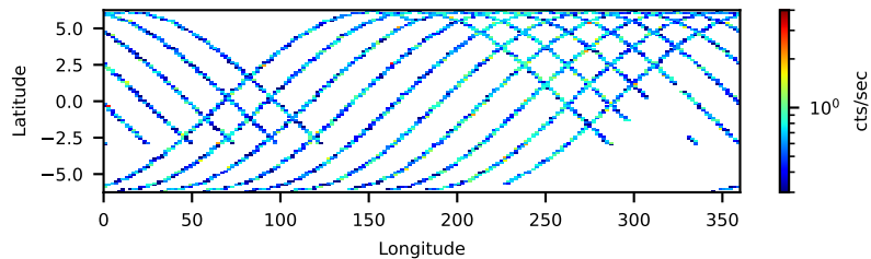
--saacalc=1 -saamode=OPTIMIZED --tentacle=no 41.03-ks, 99%
