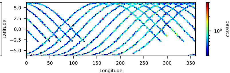
--saacalc=2 -saamode=OPTIMIZED --tentacle=no 41.17-ks, 99%
