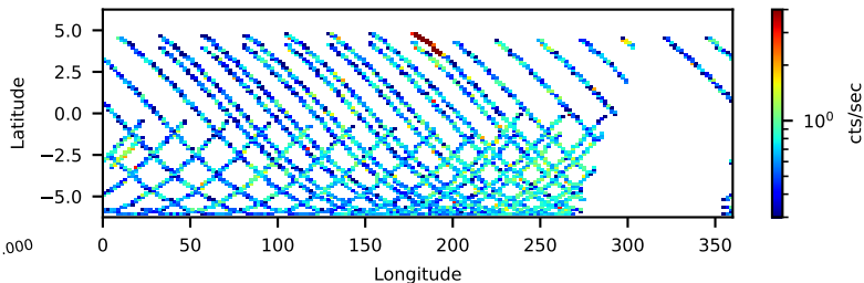
--saacalc=2 -saamode=STRICT --tentacle=yes 57.20-ks, 86%
