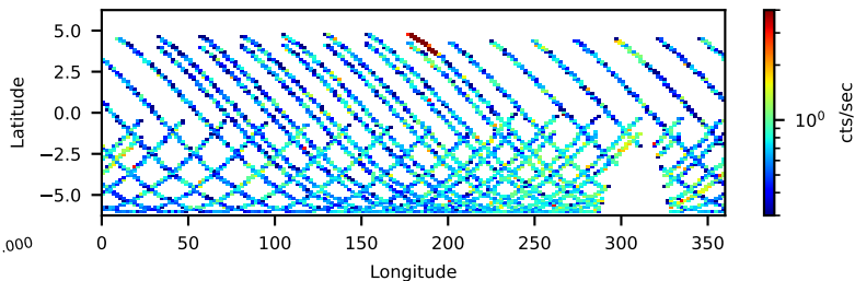
--saacalc=2 -saamode=OPTIMIZED --tentacle=yes 66.29-ks, 100%
