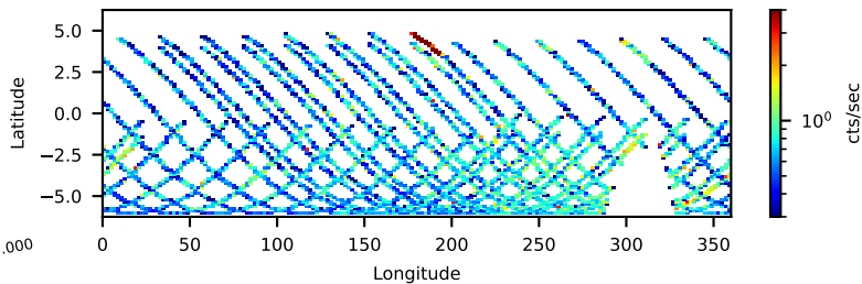
--saacalc=1 -saamode=STRICT --tentacle=no 59.87-ks, 90%
