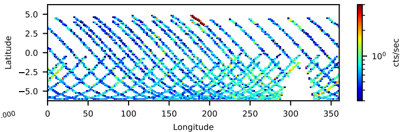
--saacalc=2 -saamode=STRICT --tentacle=no 57.20-ks, 86%
