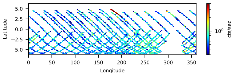
--saacalc=1 -saamode=OPTIMIZED --tentacle=yes 64.39-ks, 97%
