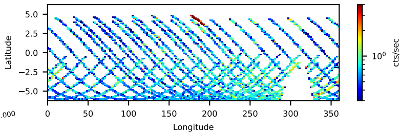
--saacalc=3 -saamode=STRICT --tentacle=no 57.20-ks, 86%
