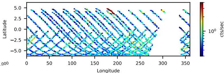
--saacalc=1 -saamode=STRICT --tentacle=yes 59.87-ks, 90%
