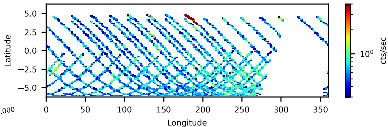
--saacalc=3 -saamode=STRICT --tentacle=yes 57.20-ks, 86%
