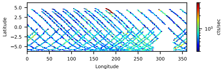
--saacalc=1 -saamode=OPTIMIZED --tentacle=no 64.39-ks, 97%
