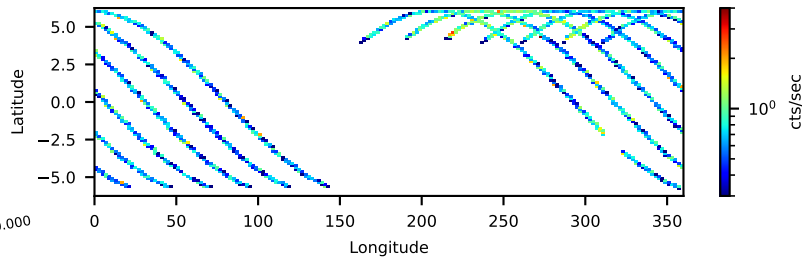
--saacalc=3 -saamode=OPTIMIZED --tentacle=no 20.82-ks, 100%
