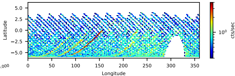
--saacalc=1 -saamode=STRICT --tentacle=no 116.90-ks, 90%
