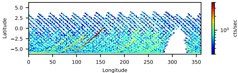
--saacalc=1 -saamode=OPTIMIZED --tentacle=yes 126.99-ks, 98%
