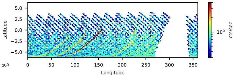
--saacalc=1 -saamode=STRICT --tentacle=yes 116.90-ks, 90%
