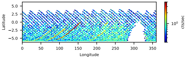
--saacalc=1 -saamode=OPTIMIZED --tentacle=no 126.99-ks, 98%
