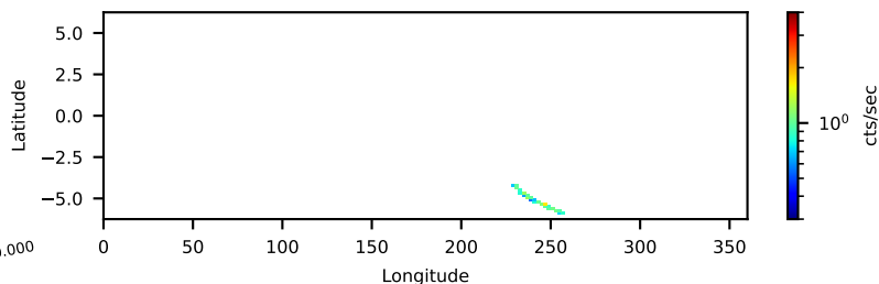
--saacalc=1 -saamode=STRICT --tentacle=yes 0.46-ks, 100%
