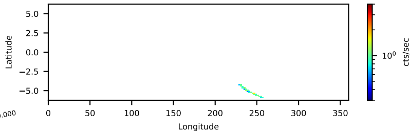
--saacalc=1 -saamode=STRICT --tentacle=no 0.46-ks, 100%
