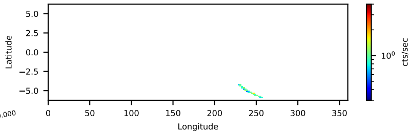
--saacalc=3 -saamode=OPTIMIZED --tentacle=no 0.46-ks, 100%
