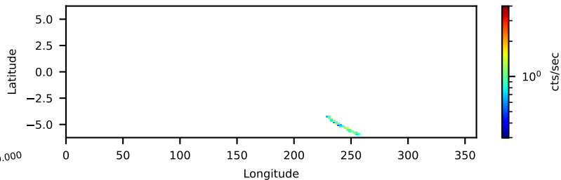
--saacalc=3 -saamode=STRICT --tentacle=yes 0.46-ks, 100%
