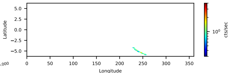
--saacalc=3 -saamode=OPTIMIZED --tentacle=yes 0.46-ks, 100%
