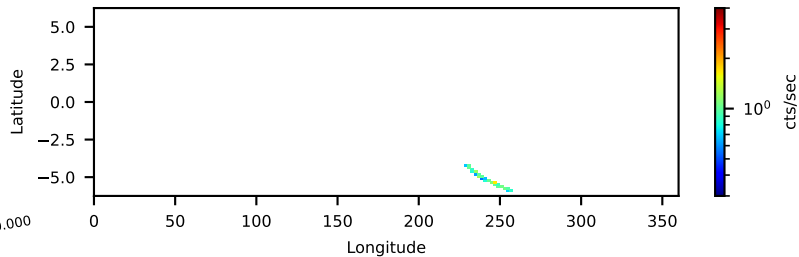
--saacalc=2 -saamode=STRICT --tentacle=no 0.46-ks, 100%
