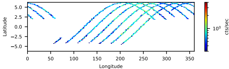
--saacalc=1 -saamode=OPTIMIZED --tentacle=yes 19.99-ks, 100%
