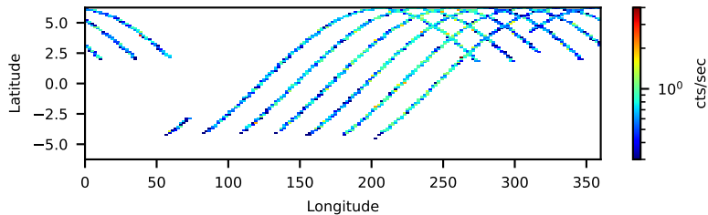
--saacalc=1 -saamode=OPTIMIZED --tentacle=no 19.99-ks, 100%
