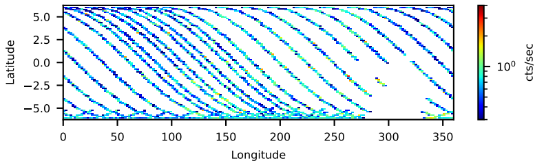
--saacalc=1 -saamode=OPTIMIZED --tentacle=yes 55.80-ks, 98%
