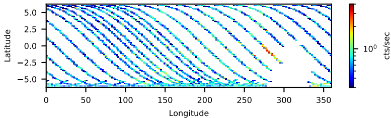
--saacalc=1 -saamode=OPTIMIZED --tentacle=no 56.08-ks, 99%
