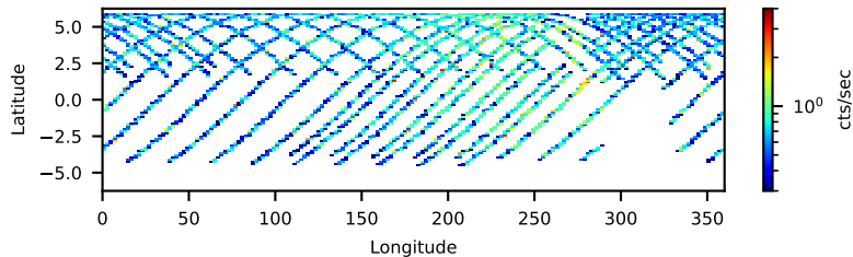
--saacalc=1 -saamode=OPTIMIZED --tentacle=yes 59.67-ks, 95%
