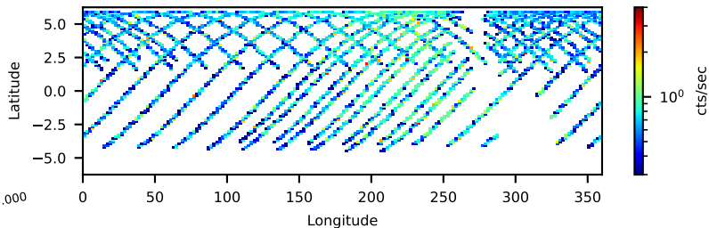
--saacalc=2 -saamode=OPTIMIZED --tentacle=yes 58.72-ks, 94%
