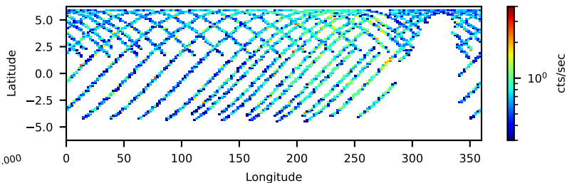
--saacalc=1 -saamode=STRICT --tentacle=yes 55.33-ks, 88%
