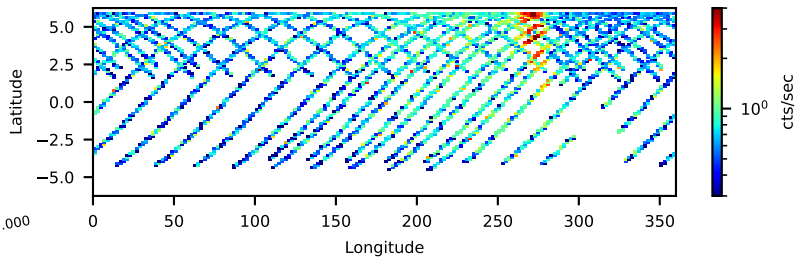
--saacalc=2 -saamode=OPTIMIZED --tentacle=no 62.51-ks, 100%
