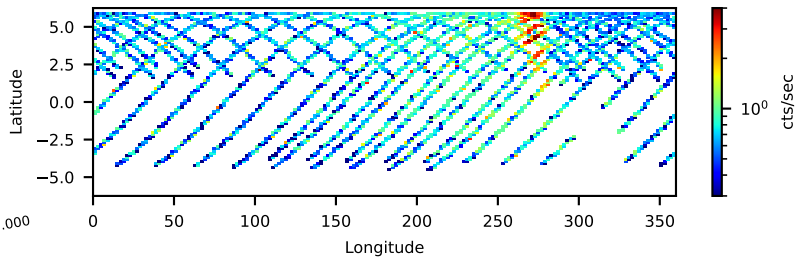
--saacalc=1 -saamode=STRICT --tentacle=no 57.88-ks, 92%
