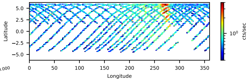
--saacalc=3 -saamode=OPTIMIZED --tentacle=no 62.51-ks, 100%
