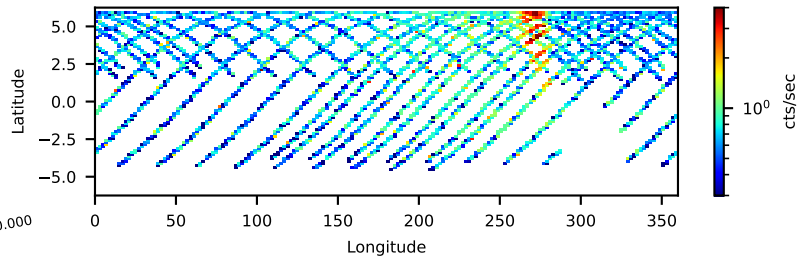
--saacalc=3 -saamode=OPTIMIZED --tentacle=yes 58.00-ks, 93%
