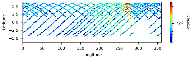
--saacalc=1 -saamode=OPTIMIZED --tentacle=no 62.23-ks, 99%
