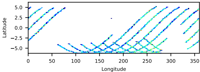
--saacalc=1 -saamode=OPTIMIZED --tentacle=no 21.94-ks, 98%
