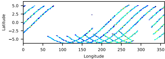
--saacalc=1 -saamode=OPTIMIZED --tentacle=yes 21.94-ks, 98%
