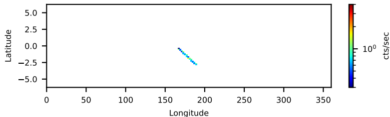
--saacalc=1 -saamode=OPTIMIZED --tentacle=yes 0.37-ks, 100%
