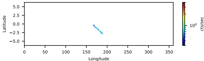
--saacalc=1 -saamode=OPTIMIZED --tentacle=no 0.37-ks, 100%
