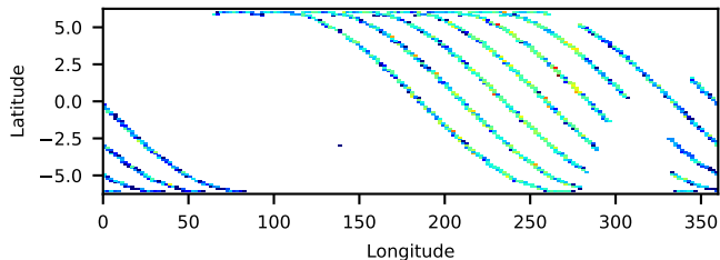
--saacalc=1 -saamode=OPTIMIZED --tentacle=yes 19.83-ks, 97%
