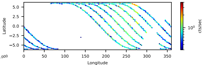
--saacalc=2 -saamode=OPTIMIZED --tentacle=no 20.45-ks, 100%
