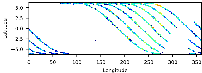
--saacalc=1 -saamode=OPTIMIZED --tentacle=no 20.09-ks, 98%
