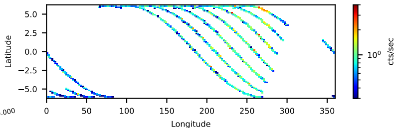
--saacalc=2 -saamode=STRICT --tentacle=yes 16.16-ks, 79%
