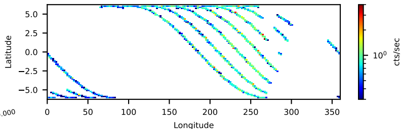
--saacalc=3 -saamode=STRICT --tentacle=yes 16.10-ks, 79%
