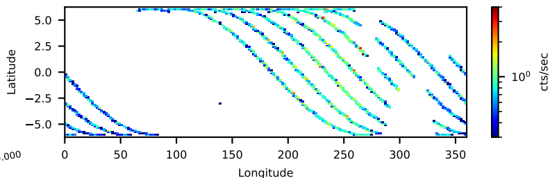
--saacalc=2 -saamode=OPTIMIZED --tentacle=yes 19.67-ks, 96%
