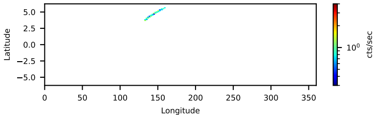
--saacalc=1 -saamode=OPTIMIZED --tentacle=yes 0.44-ks, 100%
