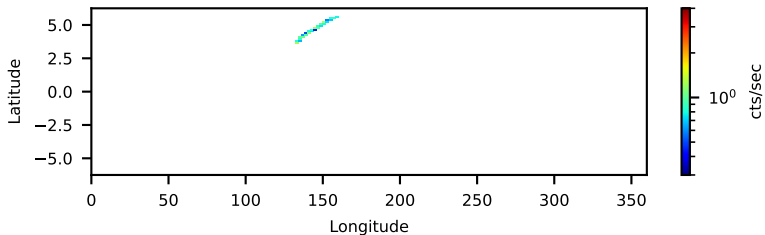
--saacalc=1 -saamode=OPTIMIZED --tentacle=no 0.44-ks, 100%
