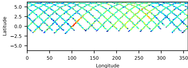
--saacalc=1 -saamode=OPTIMIZED --tentacle=yes 43.48-ks, 100%
