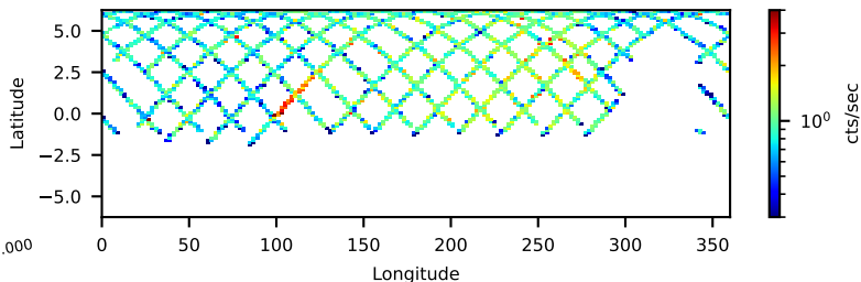
--saacalc=3 -saamode=STRICT --tentacle=yes 39.35-ks, 90%
