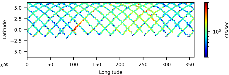
--saacalc=3 -saamode=STRICT --tentacle=no 39.35-ks, 90%
