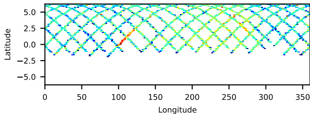
--saacalc=1 -saamode=OPTIMIZED --tentacle=no 43.48-ks, 100%
