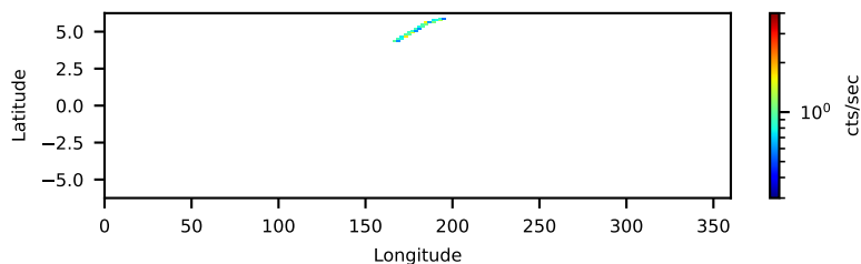
--saacalc=1 -saamode=OPTIMIZED --tentacle=yes 0.46-ks, 100%
