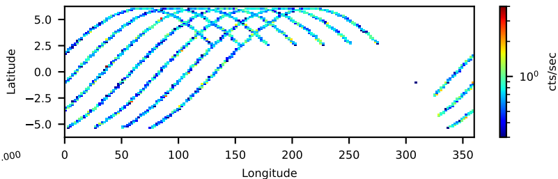
--saacalc=2 -saamode=OPTIMIZED --tentacle=yes 21.64-ks, 100%
