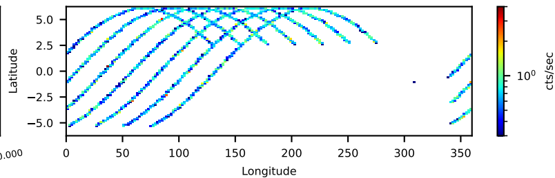
--saacalc=1 -saamode=STRICT --tentacle=yes 21.15-ks, 98%
