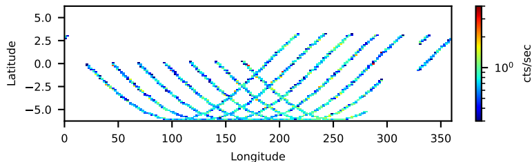
--saacalc=1 -saamode=OPTIMIZED --tentacle=yes 20.72-ks, 97%
