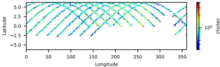
--saacalc=1 -saamode=OPTIMIZED --tentacle=no 29.91-ks, 98%
