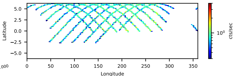
--saacalc=3 -saamode=STRICT --tentacle=yes 26.05-ks, 85%
