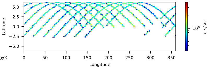
--saacalc=3 -saamode=STRICT --tentacle=no 26.05-ks, 85%
