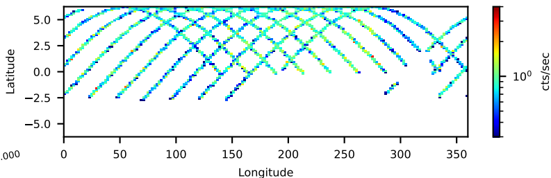
--saacalc=3 -saamode=OPTIMIZED --tentacle=yes 30.47-ks, 100%
