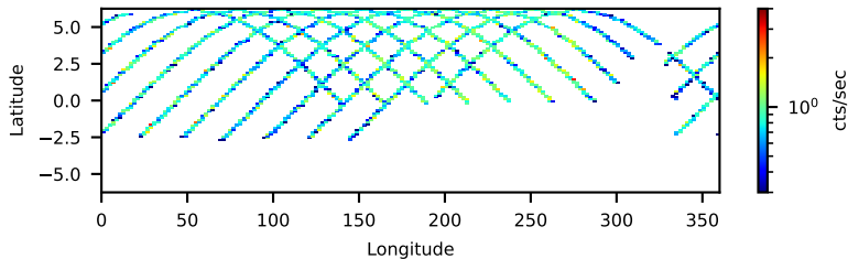
--saacalc=1 -saamode=OPTIMIZED --tentacle=yes 29.91-ks, 98%
