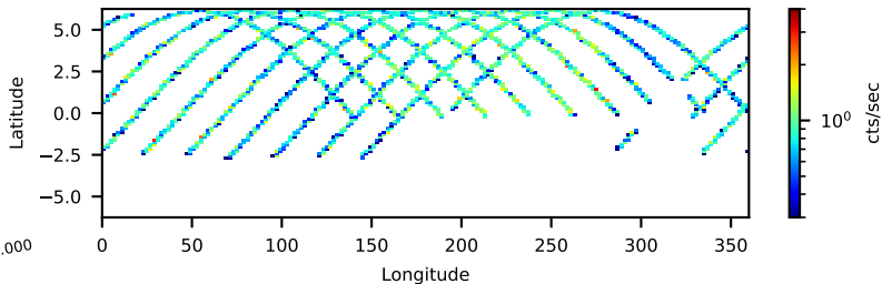
--saacalc=3 -saamode=OPTIMIZED --tentacle=no 30.47-ks, 100%
