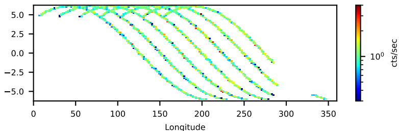
--saacalc=2 -saamode=OPTIMIZED --tentacle=yes 20.68-ks, 99%
