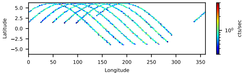
--saacalc=1 -saamode=OPTIMIZED --tentacle=yes 20.53-ks, 99%
