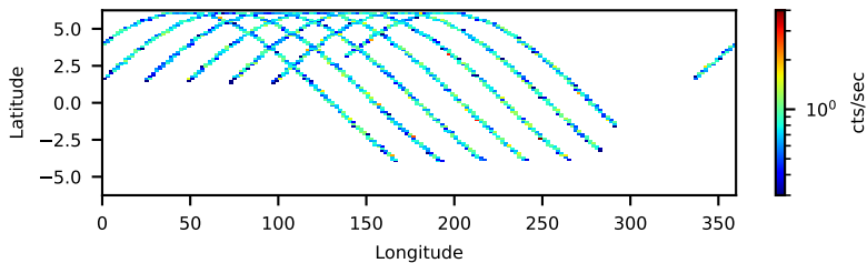
--saacalc=1 -saamode=OPTIMIZED --tentacle=no 20.53-ks, 99%
