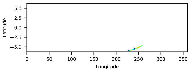
--saacalc=1 -saamode=OPTIMIZED --tentacle=yes 0.49-ks, 100%
