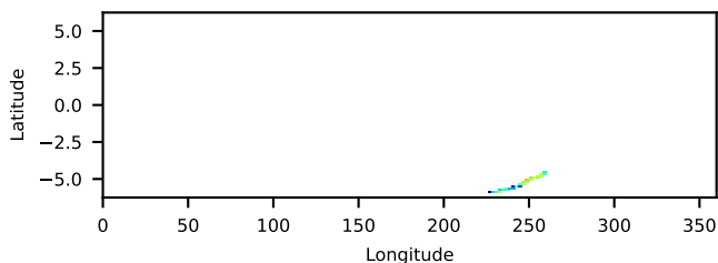
--saacalc=1 -saamode=OPTIMIZED --tentacle=no 0.49-ks, 100%
