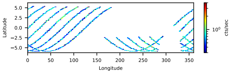
--saacalc=1 --saamode=OPTIMIZED --tentacle=no 21.54-ks, 97%
