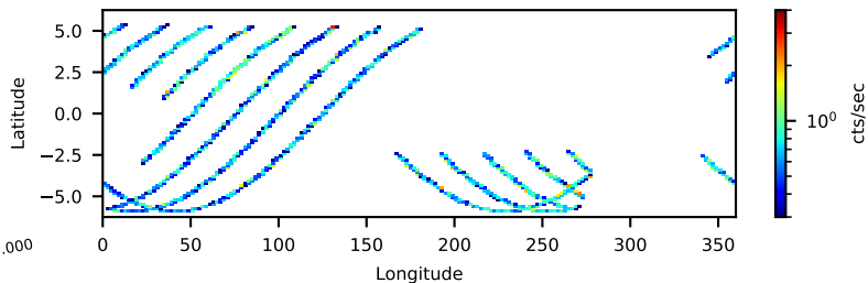
--saacalc=2 --saamode=STRICT --tentacle=yes 16.31-ks, 74%
