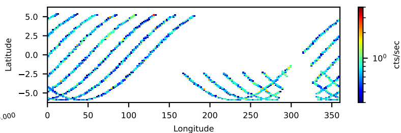
--saacalc=2 --saamode=STRICT --tentacle=no 16.31-ks, 74%
