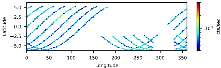
--saacalc=1 --saamode=OPTIMIZED --tentacle=yes 21.54-ks, 97%
