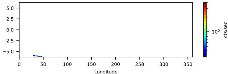
--saacalc=3 -saamode=STRICT --tentacle=yes 0.28-ks, 100%
