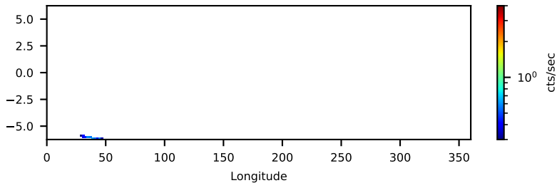
--saacalc=2 -saamode=STRICT --tentacle=no 0.28-ks, 100%
