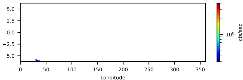
--saacalc=1 -saamode=STRICT --tentacle=yes 0.28-ks, 100%
