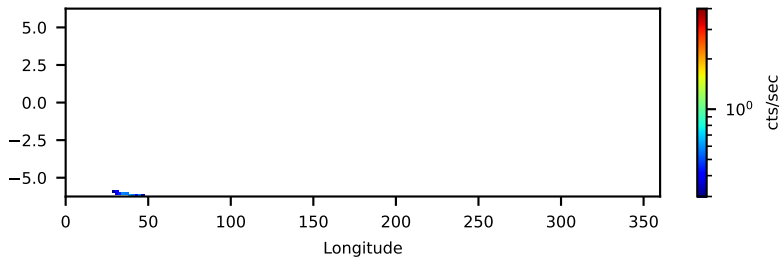
--saacalc=2 -saamode=STRICT --tentacle=yes 0.28-ks, 100%
