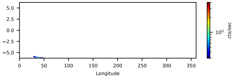
--saacalc=3 -saamode=STRICT --tentacle=no 0.28-ks, 100%
